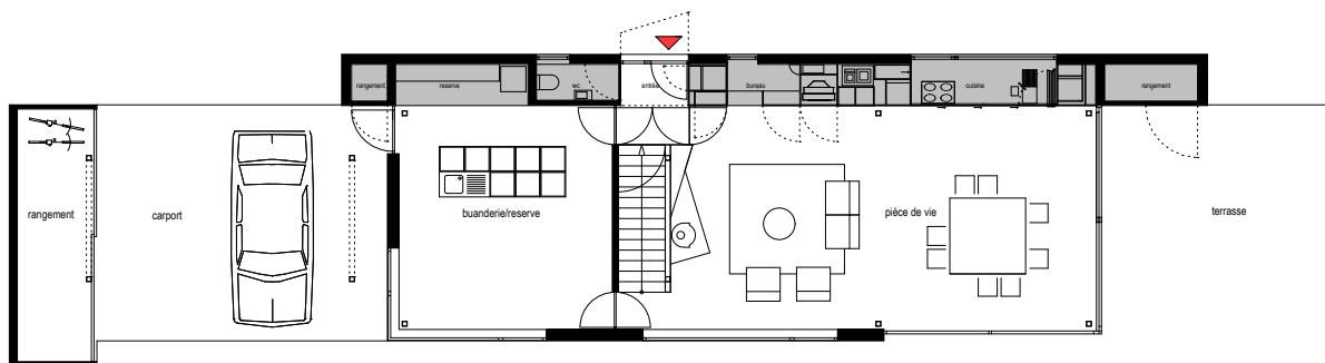
vue en plan R0 1/200
